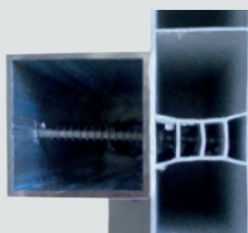
Lame PVC alvéolée renforcée
